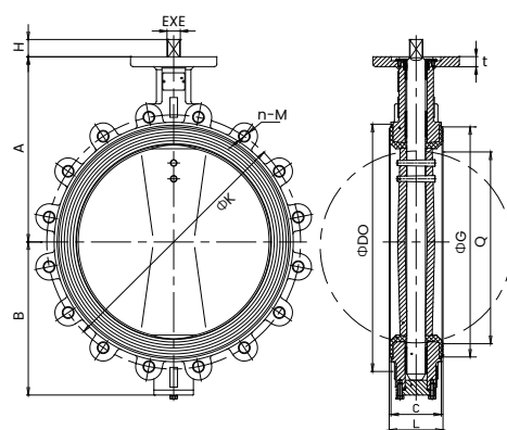
DN400-600
