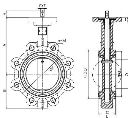
DN50-350
